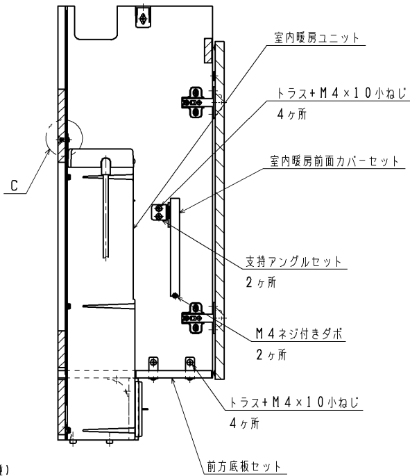
室内暖房ユニット固定詳細
