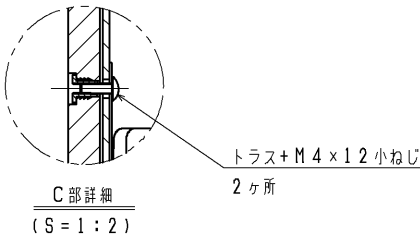
室内暖房ユニット固定詳細
