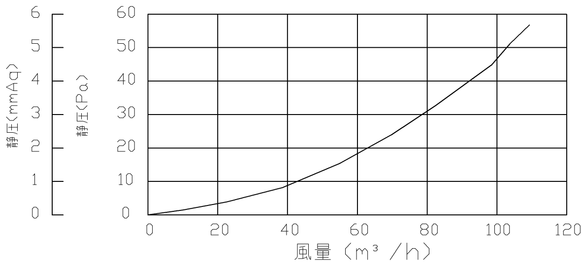
圧力損失曲線
