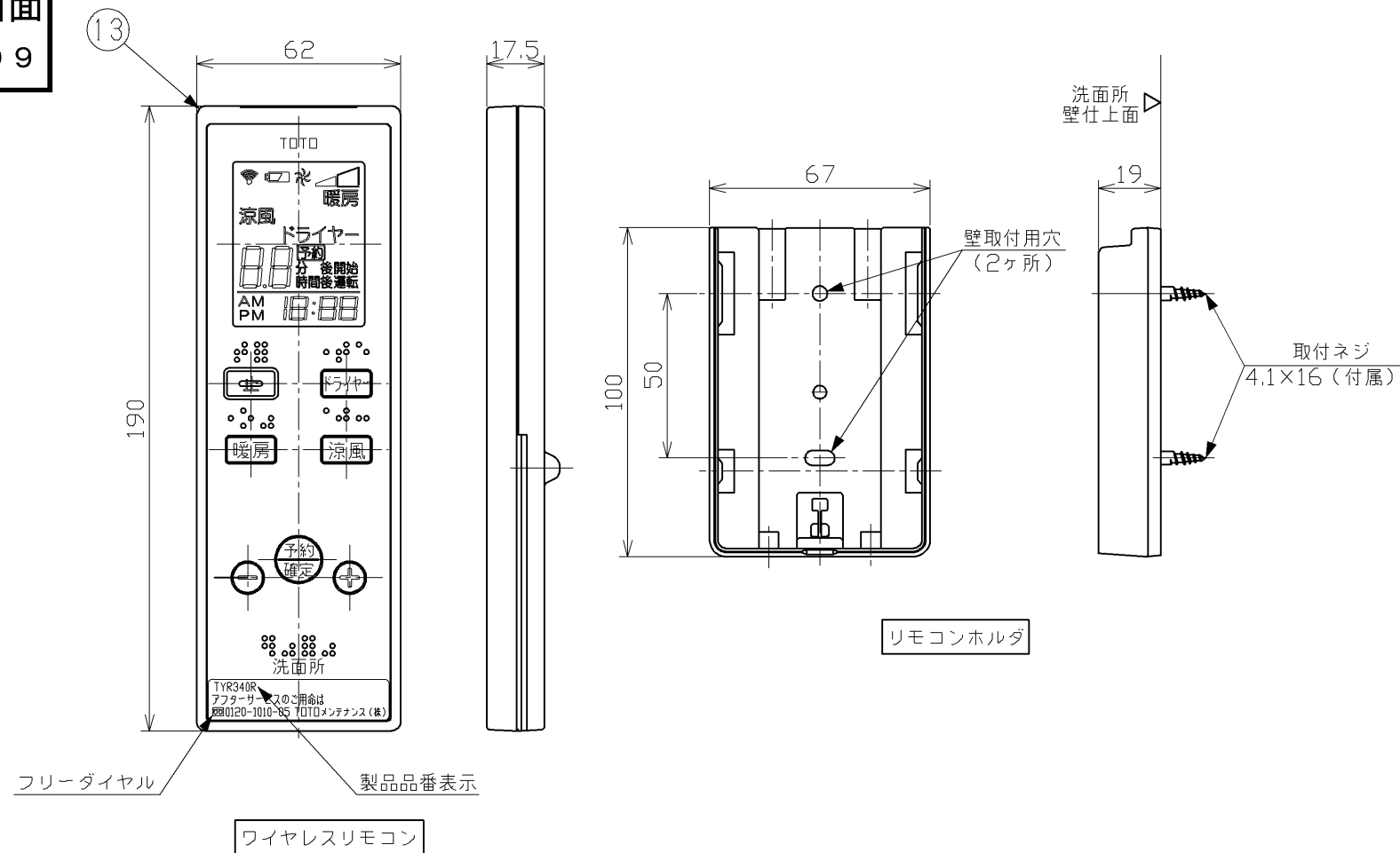
リモコン組品外観（1：2）
