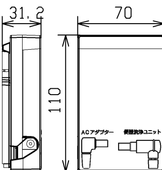
受信(ユニット)
