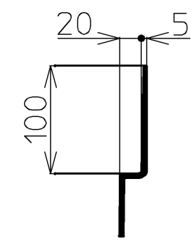
壁のせ部(防水リム部)詳細
