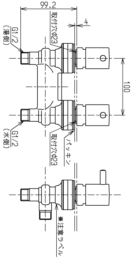
バルブ部詳細
