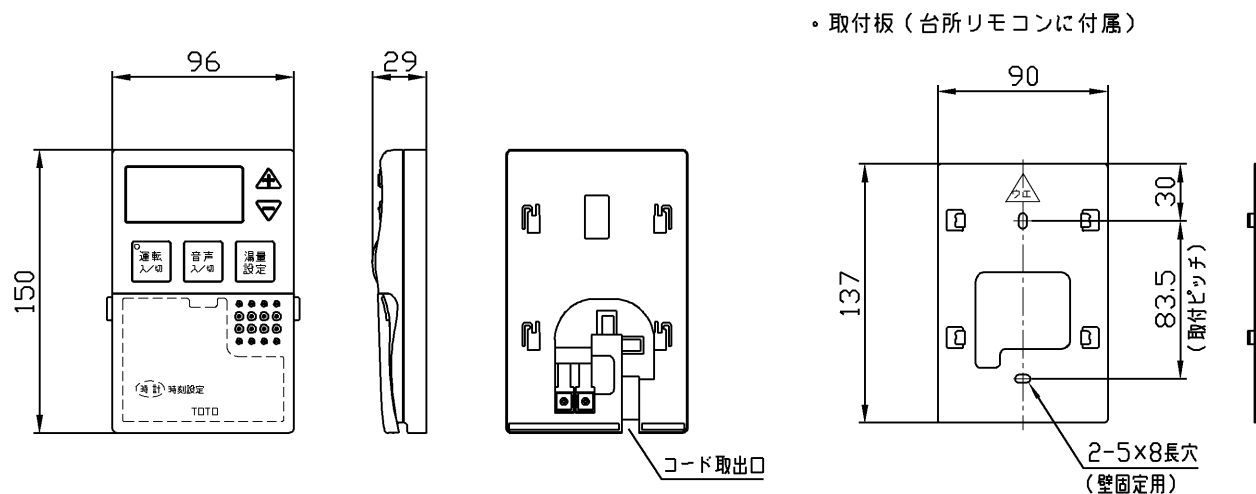
■ 台所リモコン（別売品：RAC134K） （1：4）
