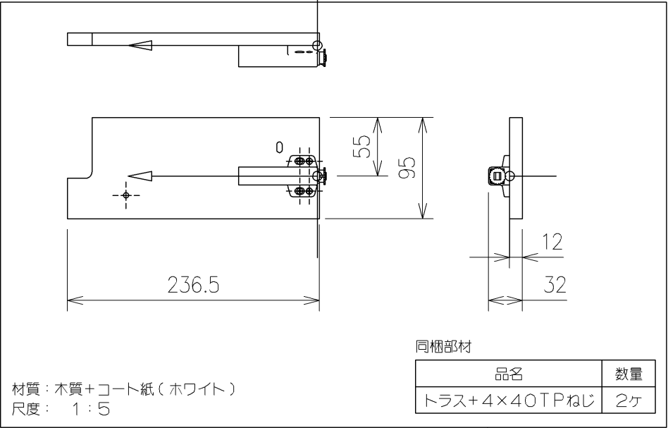
側板組品
