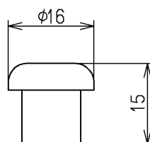
ゴムワッシャー(1:1)
