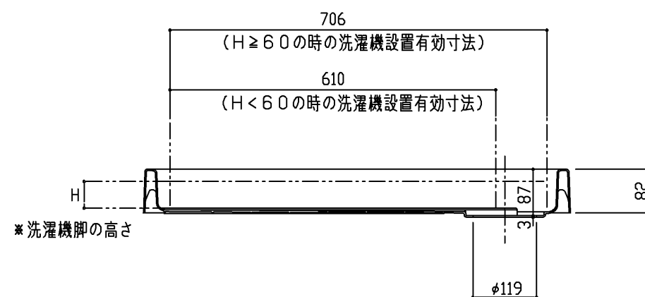
断面A-A
