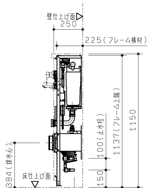
R 視図
