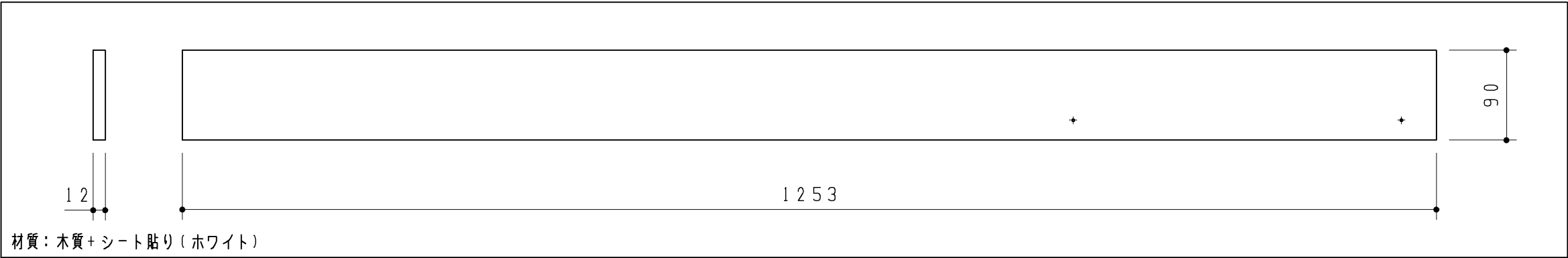
上段補強板
