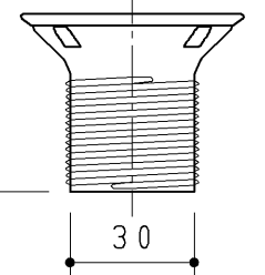
排水金具
