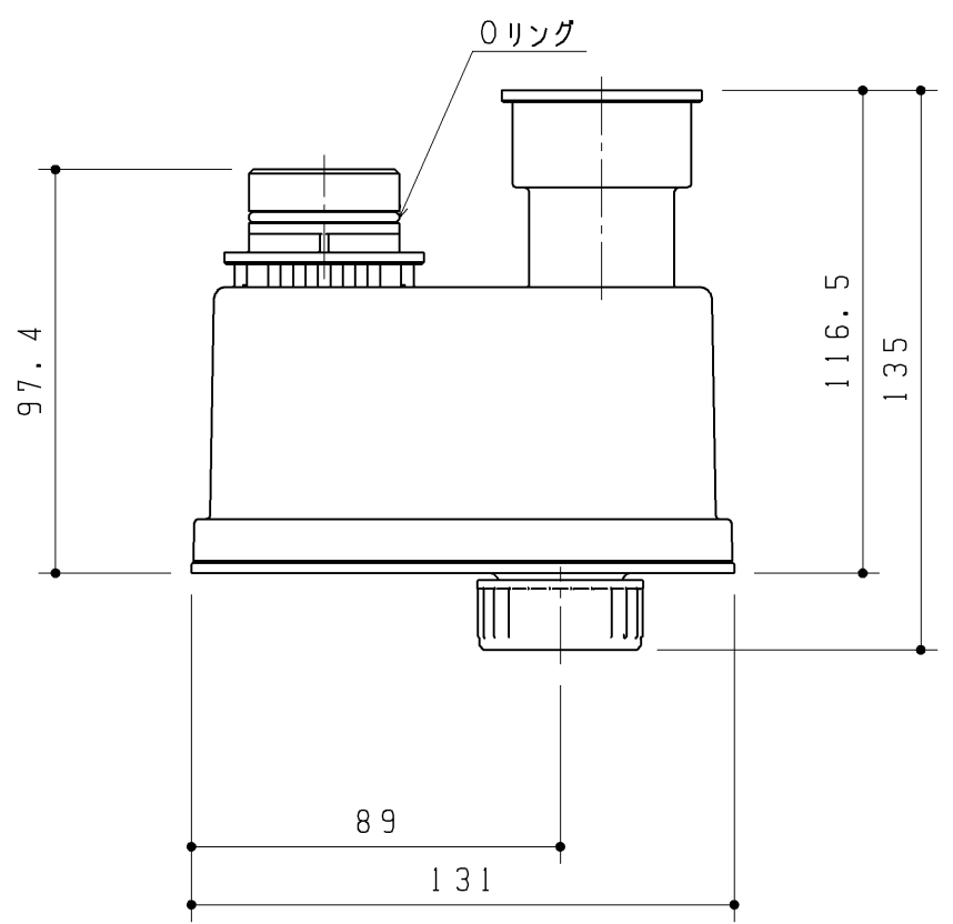
ドラムトラップ (掃除口付)
