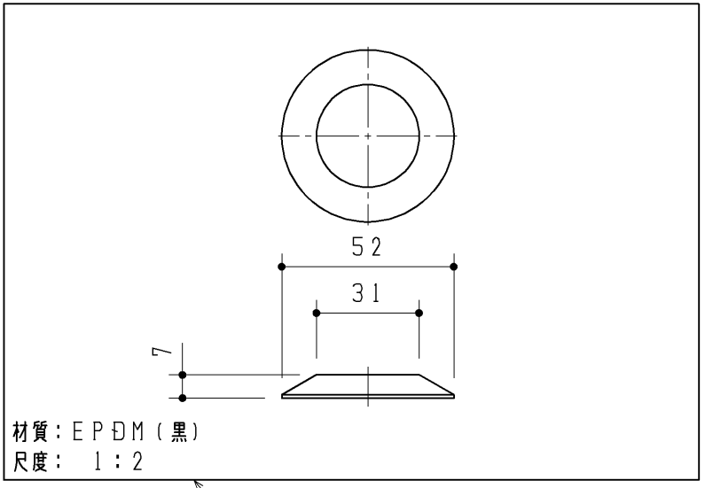
三角パッキン
