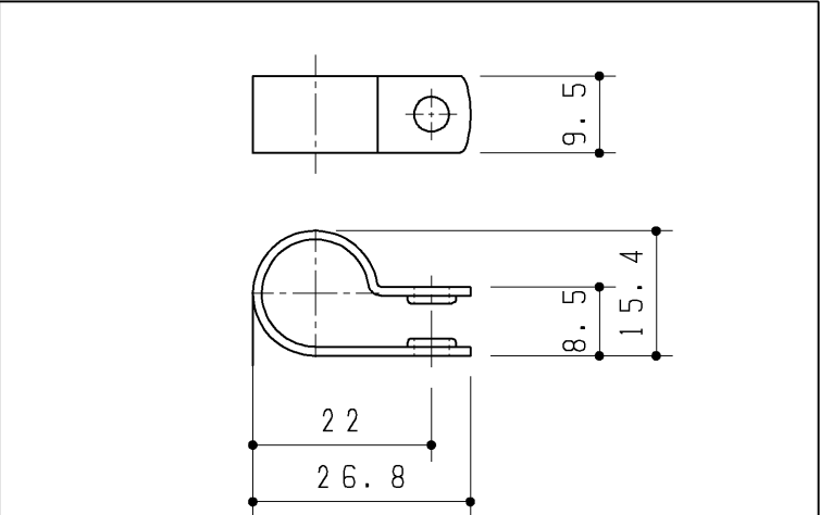
ホースクランプ (3ヶ)
