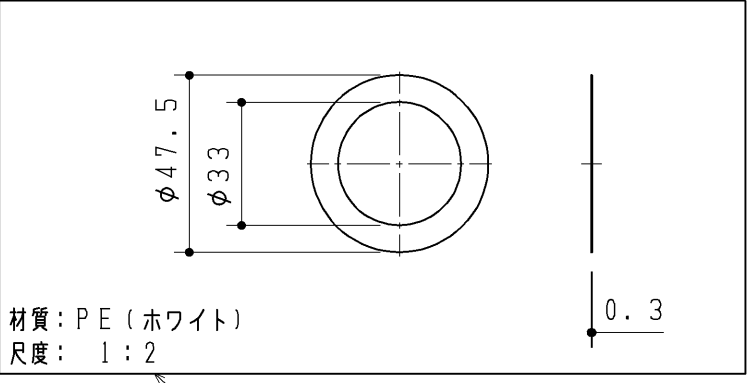
手洗器排水用スリップワッシャ
