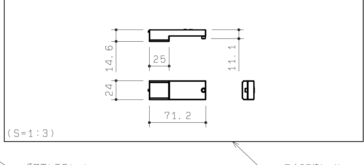
便器下LEDセット
