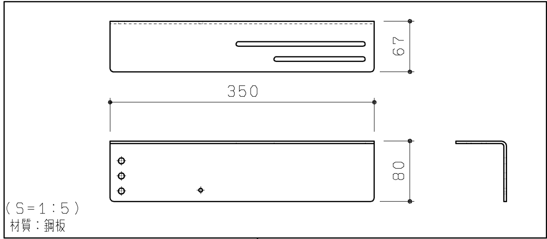
間口調整材L
