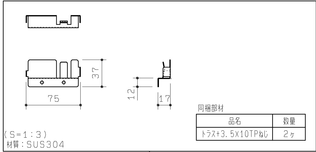
マイクロ波センサ取付金具セット
