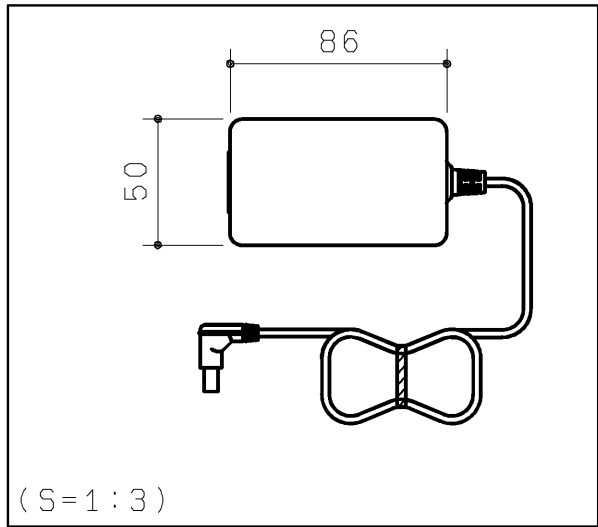
ACアダプター
