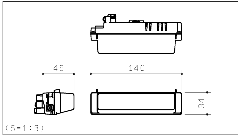
便器下LEDユニット
