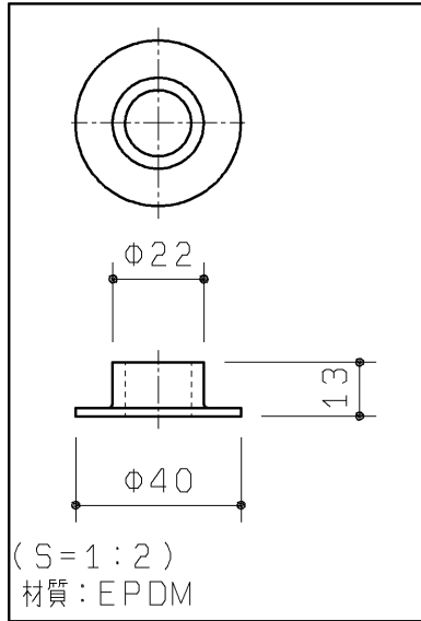
異形ゴムパッキン (2ヶ)
