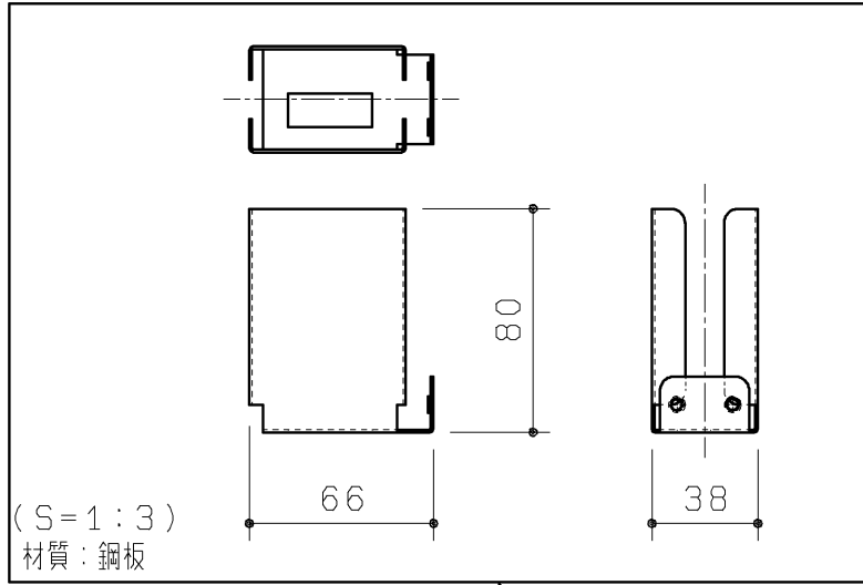
ACアダプタ取付金具
