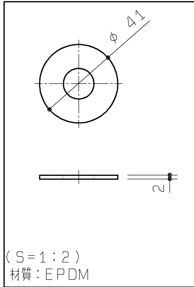
平ゴムパッキン (2ヶ)
