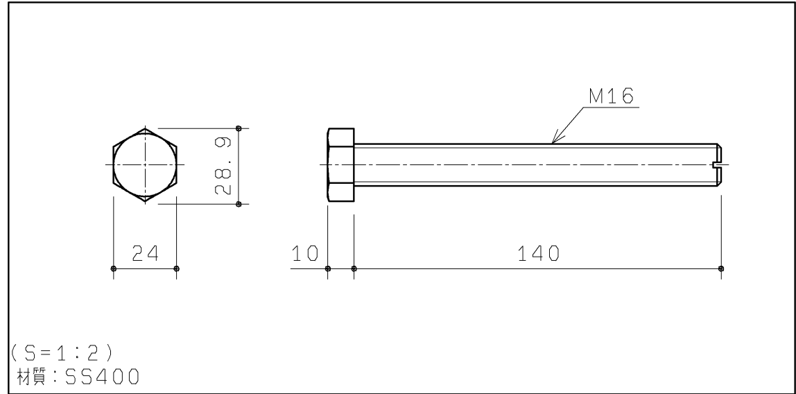
六角全ねじボルトM16X140 (2ヶ)
