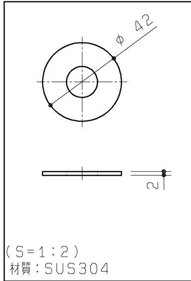
化粧座金M16 (4ヶ)
