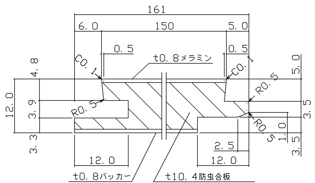
A-A断面図(1:1)
