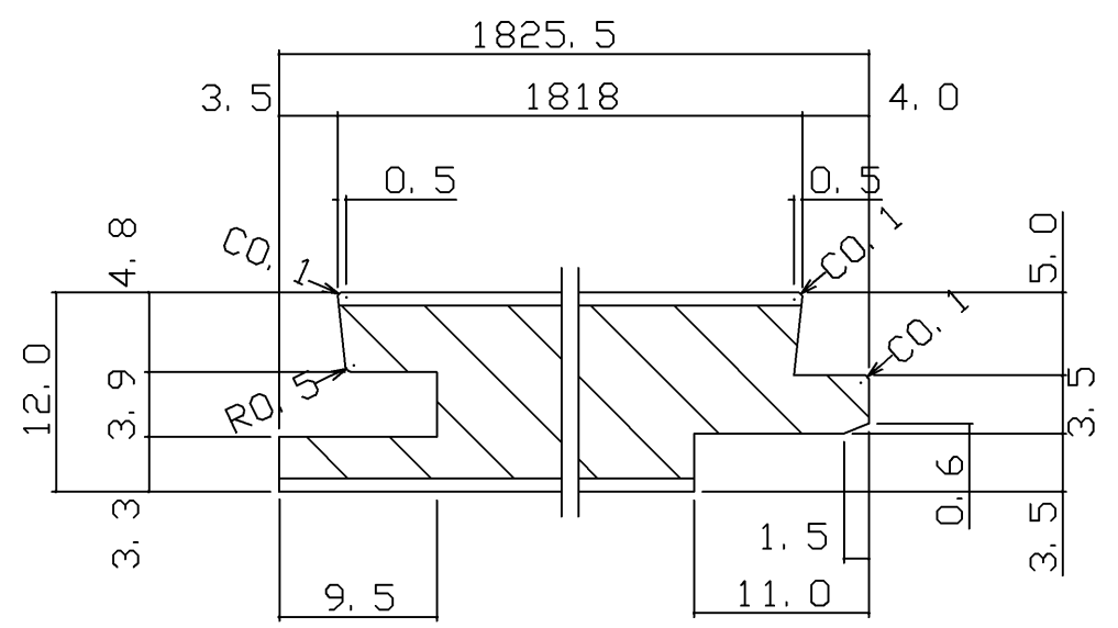
B-B断面図(1:1)
