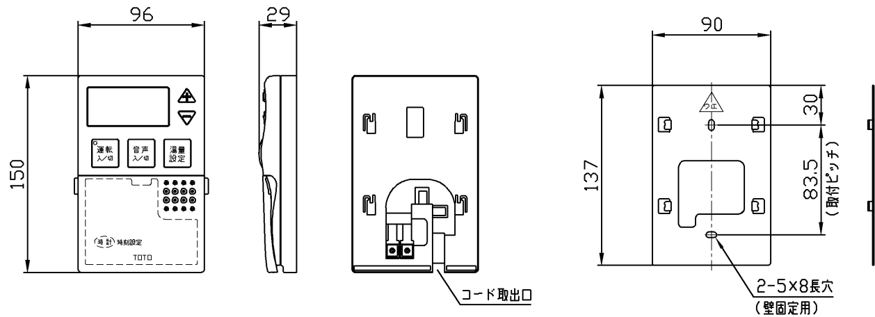
■ 台所リモコン（別売品：RAC134K） （1：4）
