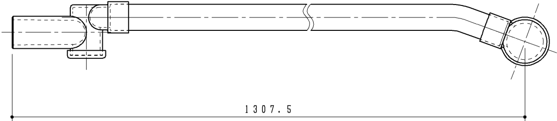
配管カバー (L=885)
