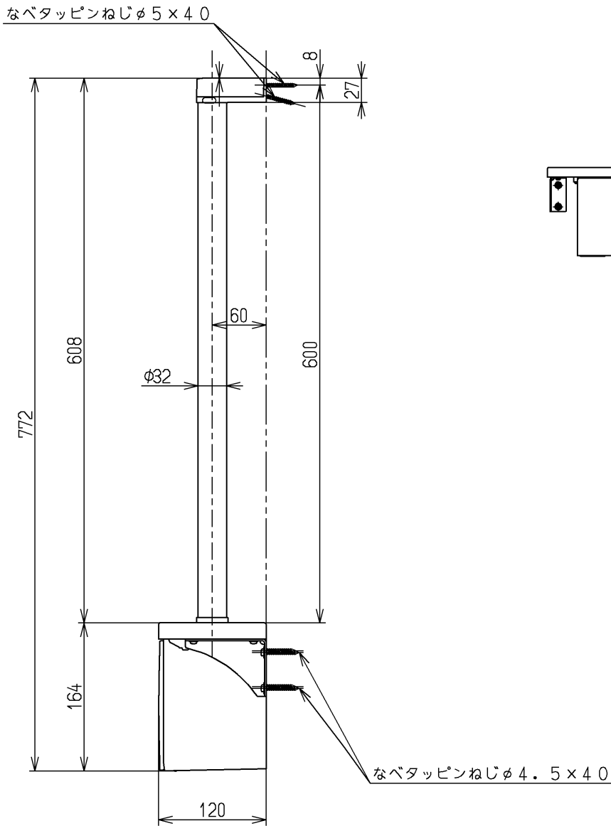
右壁設置の場合(1:10)
