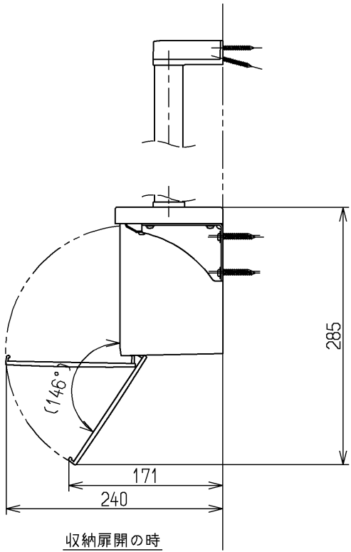
右壁設置の場合(1:10)
