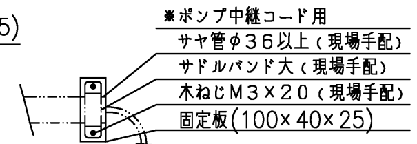
サヤ管固定部詳細図
