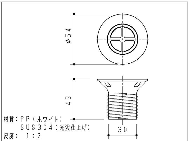
排水金具
