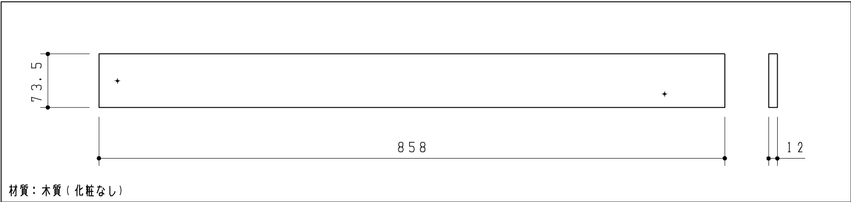
下段補強板
