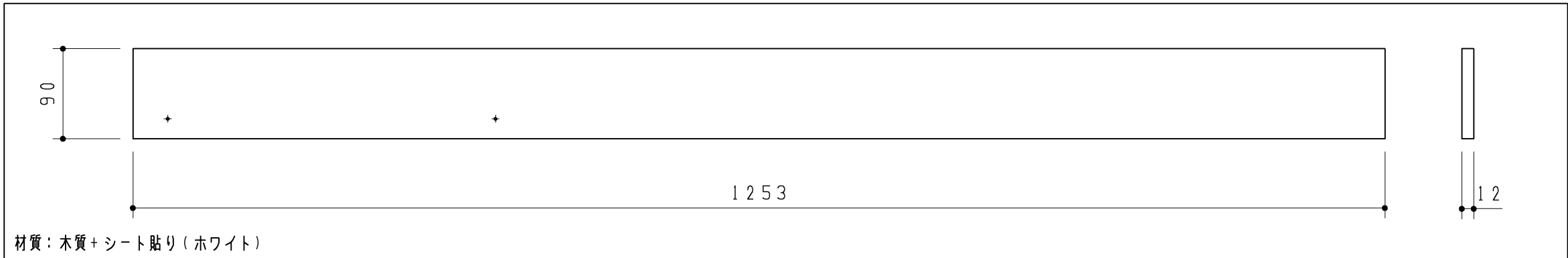
上段補強板
