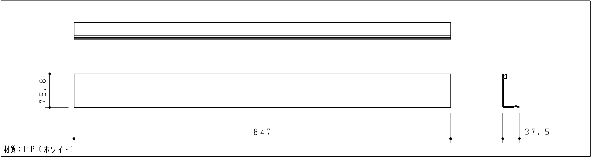
配管カバー
