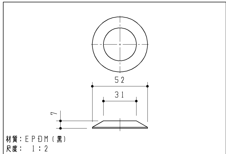
三角パッキン
