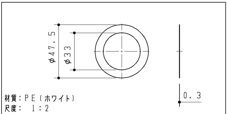
手洗器排水用スリップワッシャー
