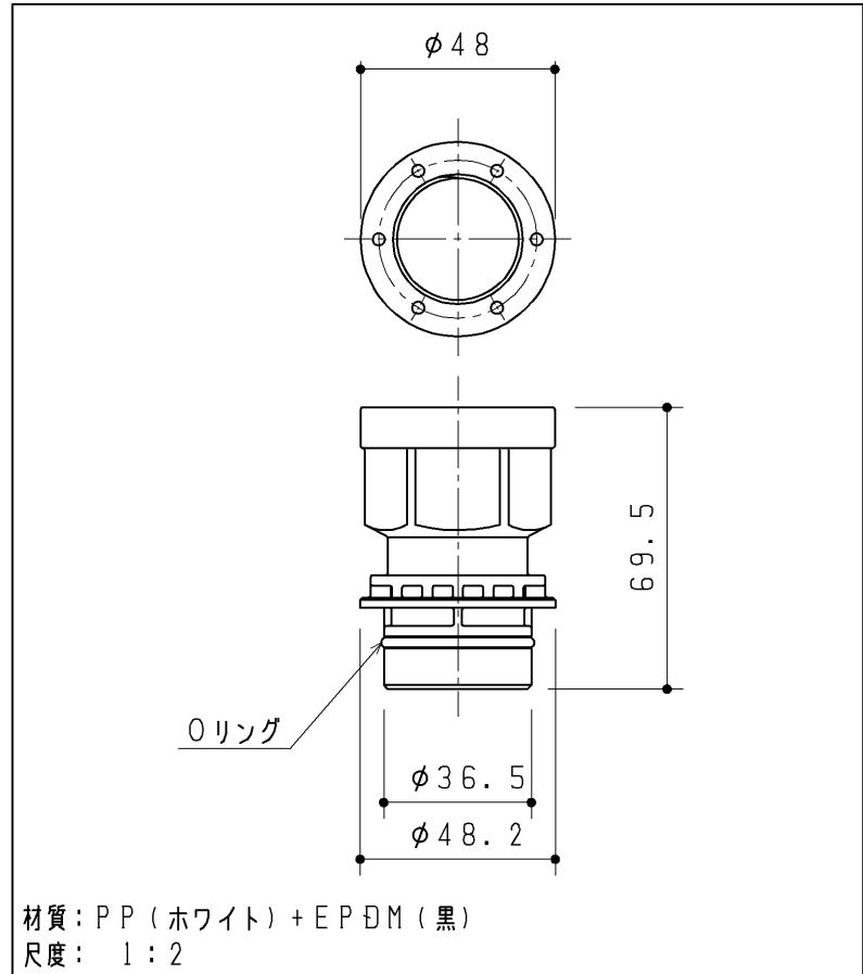
トラップ接続管
