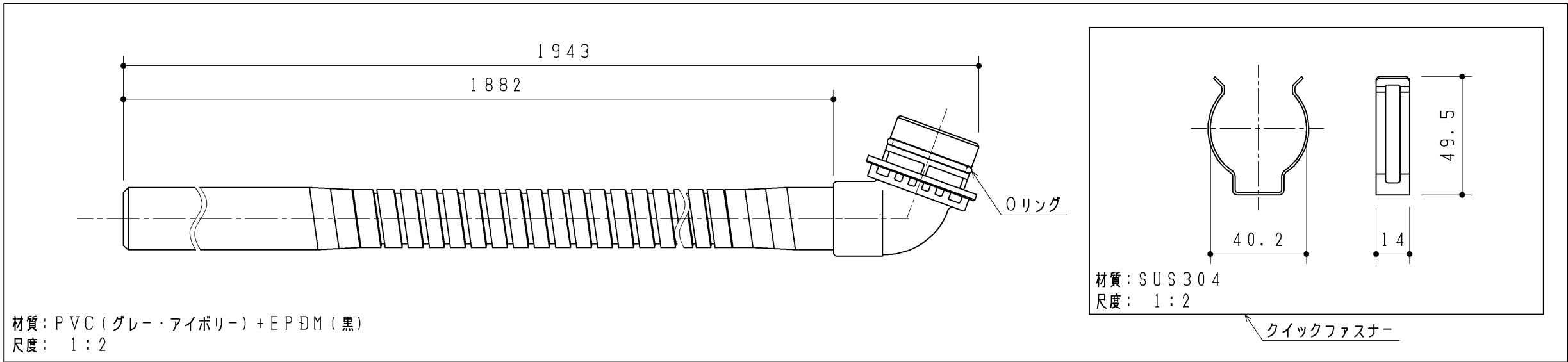
手洗排水ホースセット
