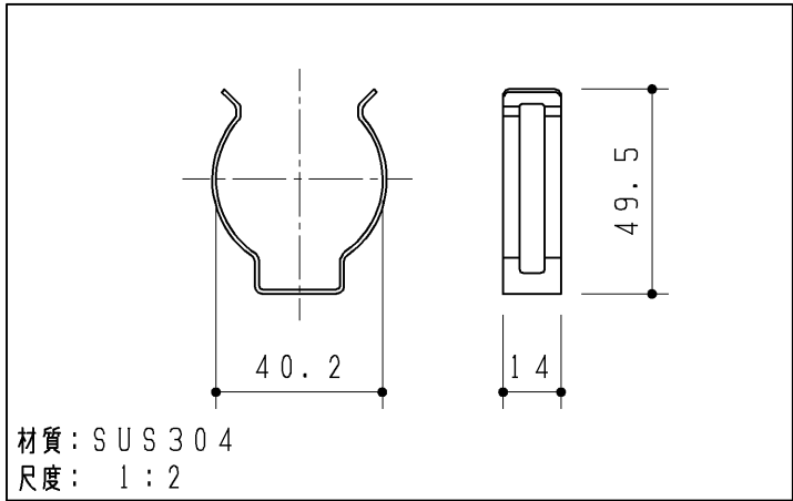
クイックファスナー
