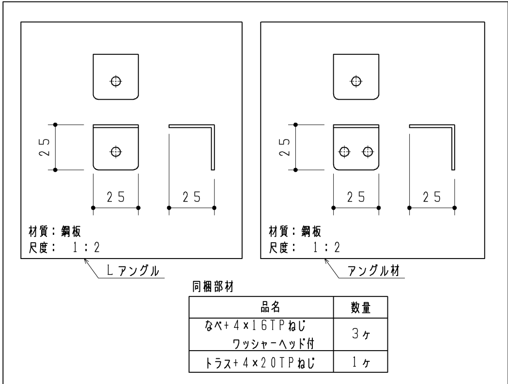
カウンター固定アングルセット
