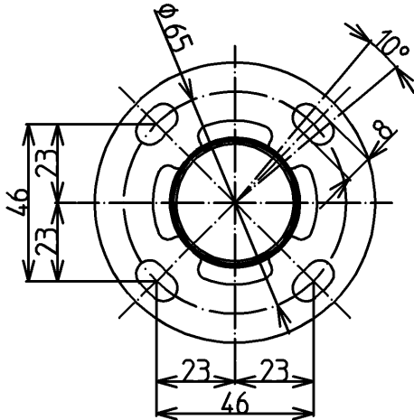
取付座詳細(1:2)
