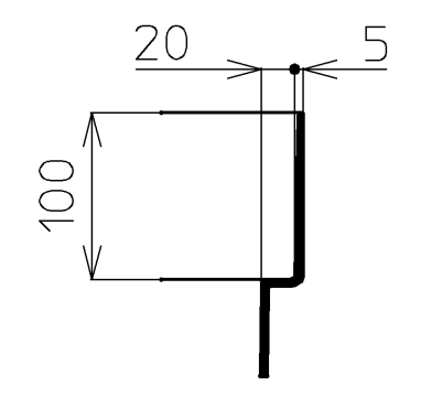
壁のせ部(防水リム部)詳細
