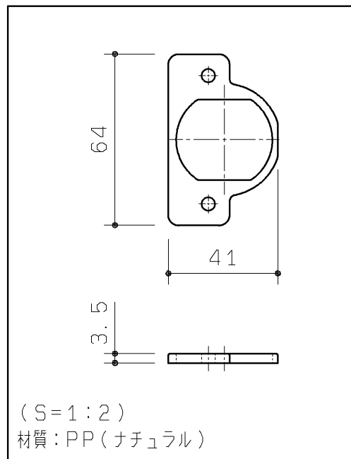
丁番用スペーサー(2ヶ)
