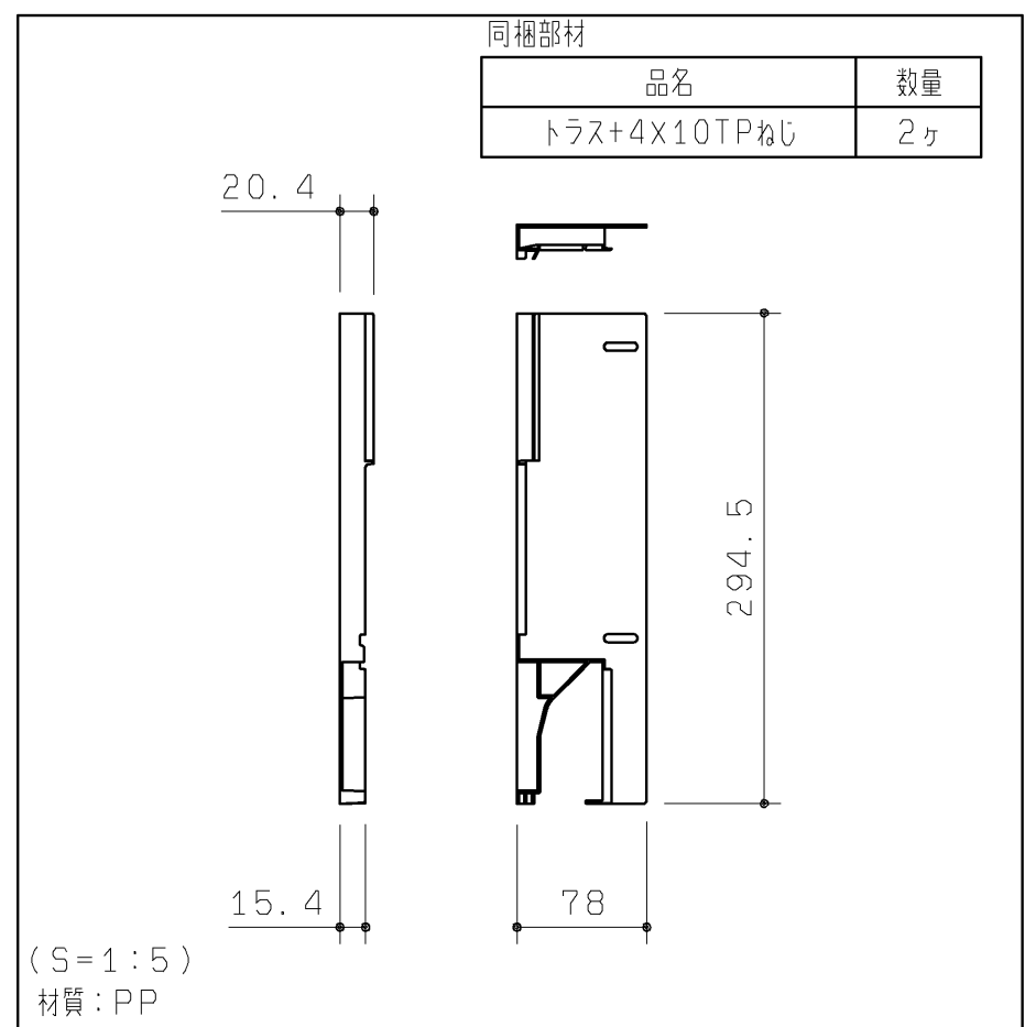
固定扉キャップセット
