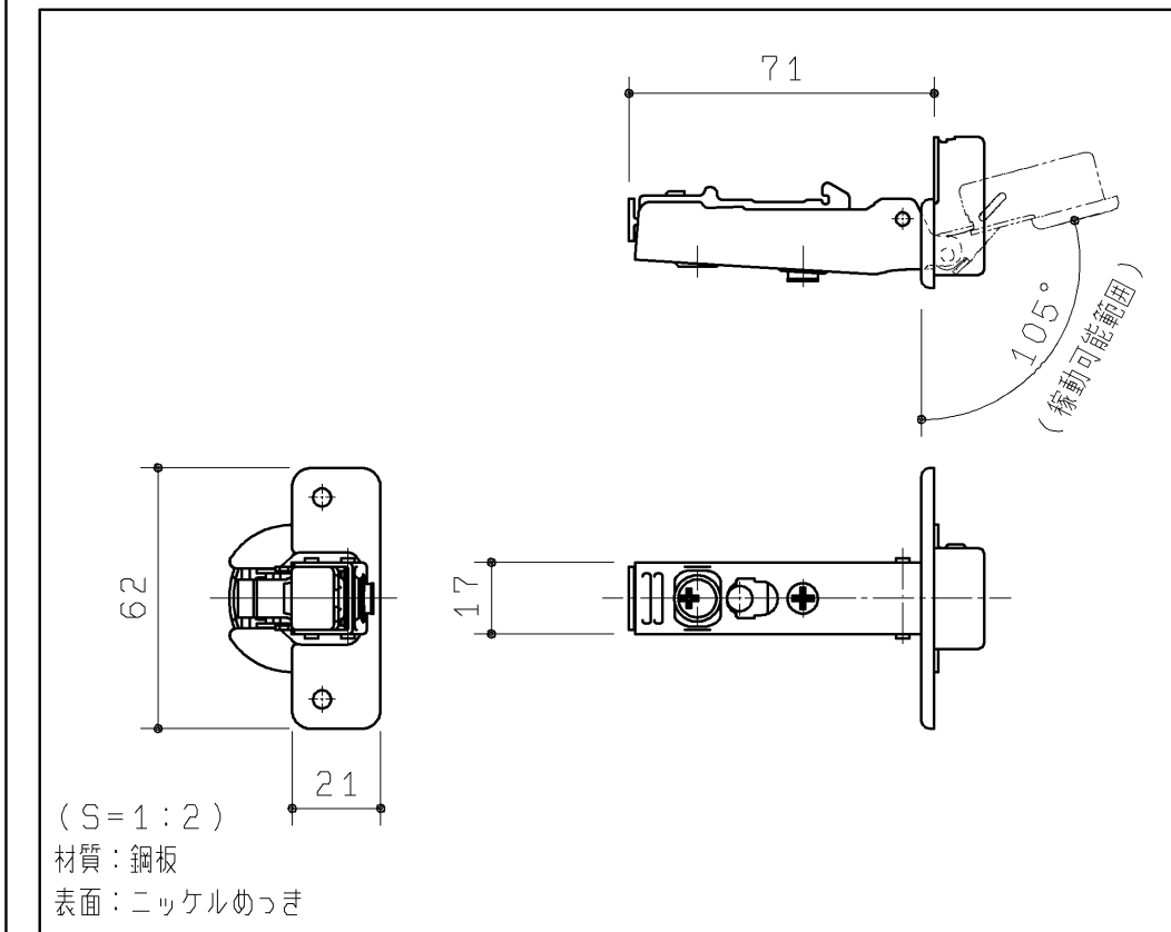
ワンタッチスライド丁番(2ヶ)
