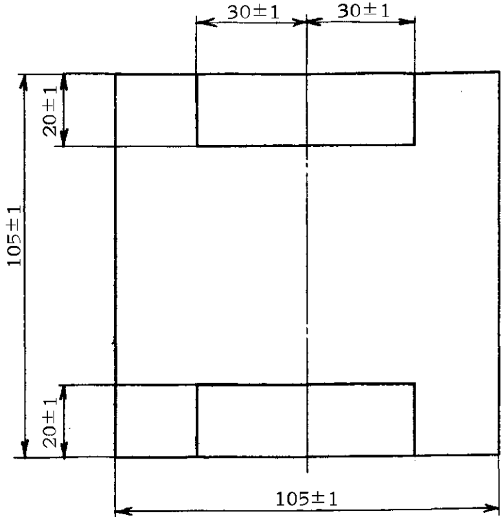
パネル壁ノ穴開ケ加工寸法
