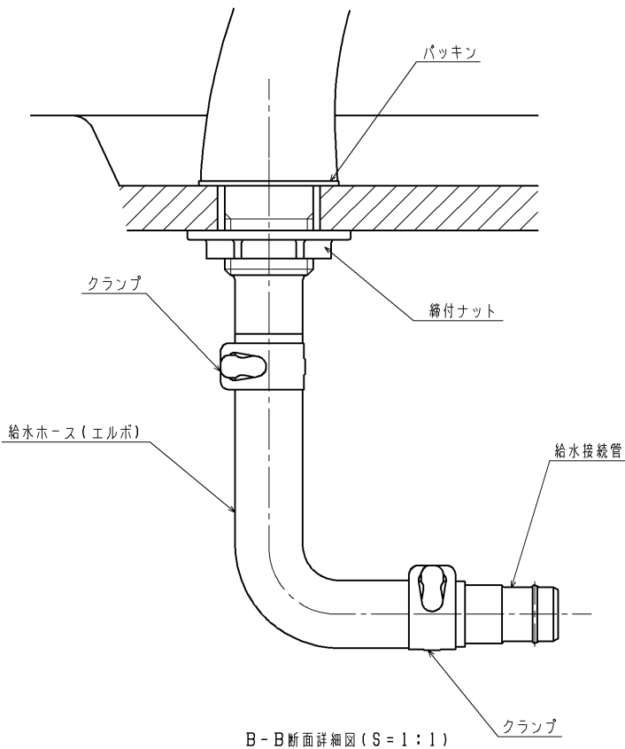
B-B断面詳細図(S=1:1)
