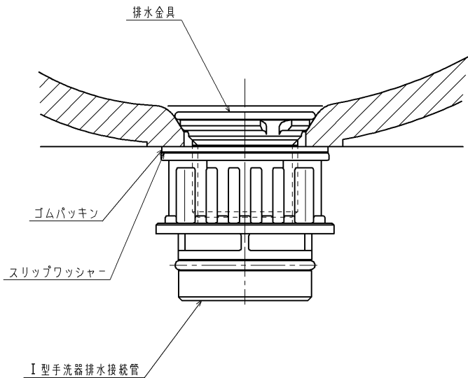
A-A断面詳細図(S=1:1)
