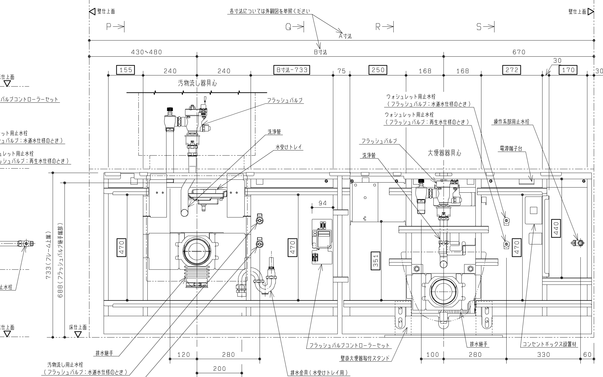
S 視図
