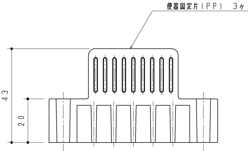
A - A 断面図
