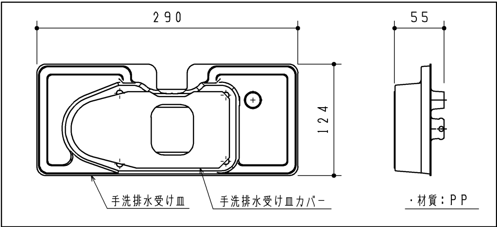
排水受け皿
