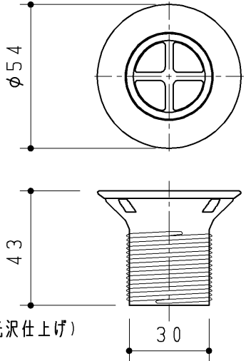
排水金具
