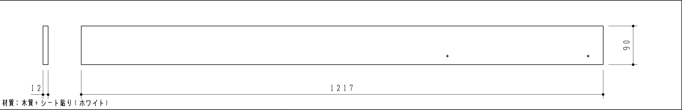
上段補強桟
