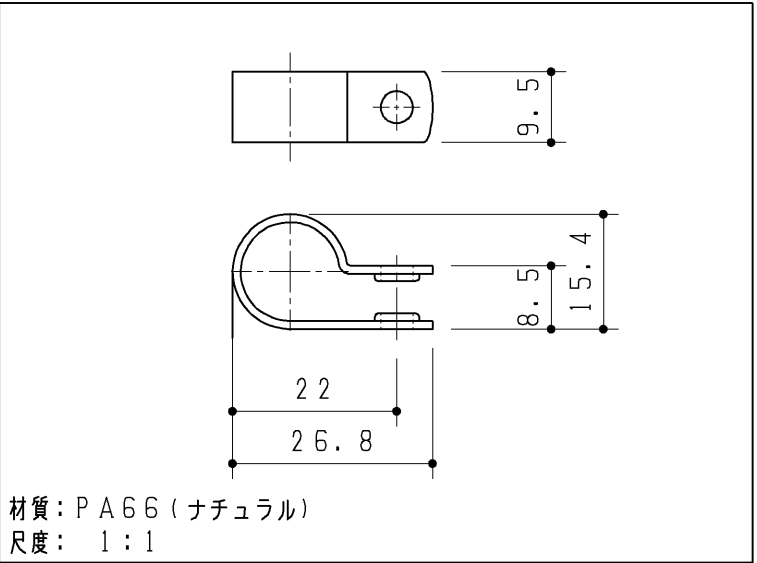
ホースクランプ (3ヶ)
