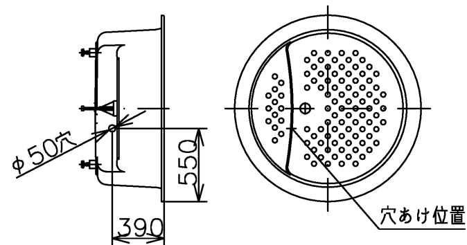
追焚用穴あけ可能位置(1:40)
