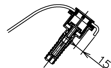
断面A-A(1:5)
