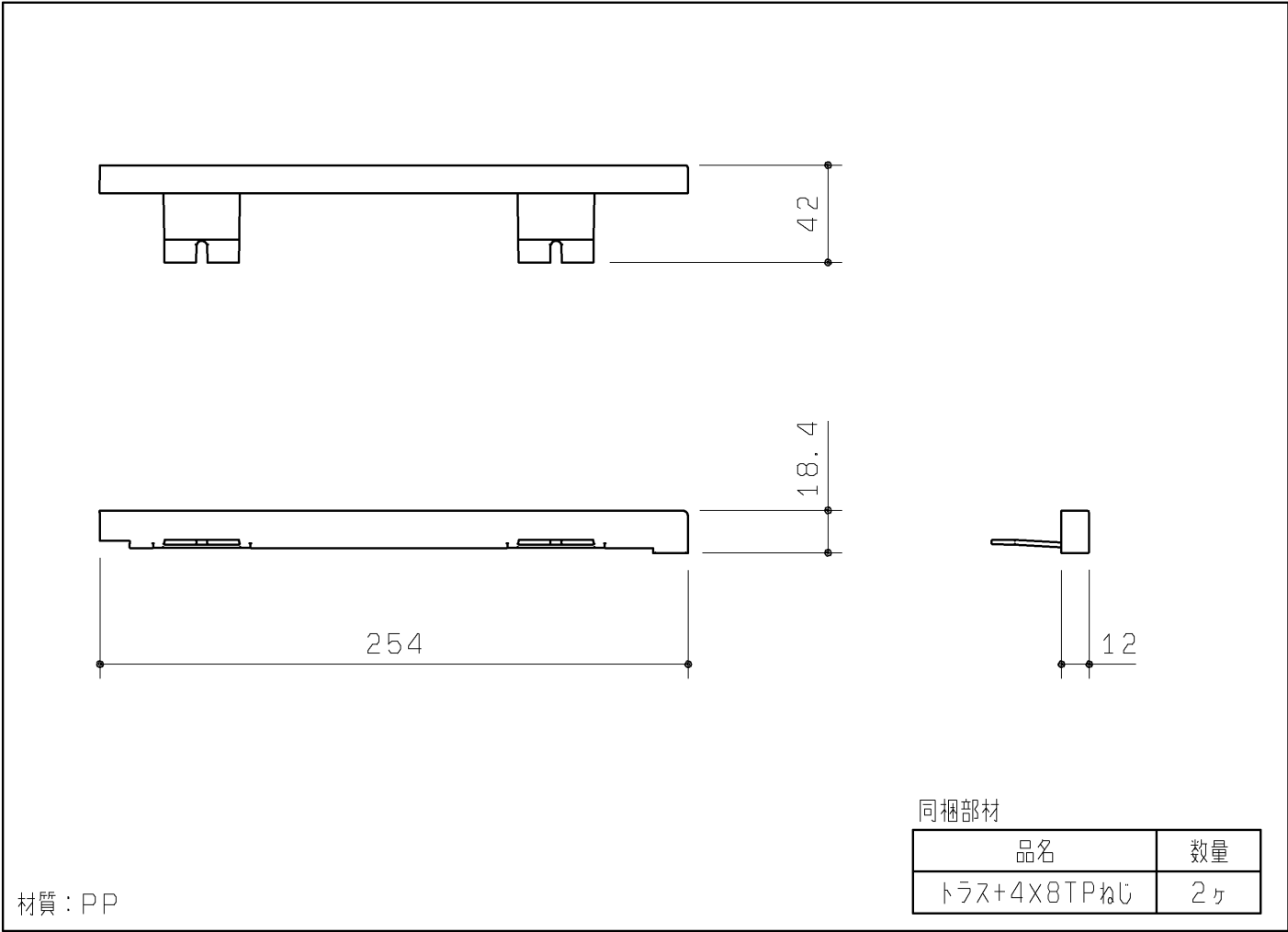
天板キャップセット
