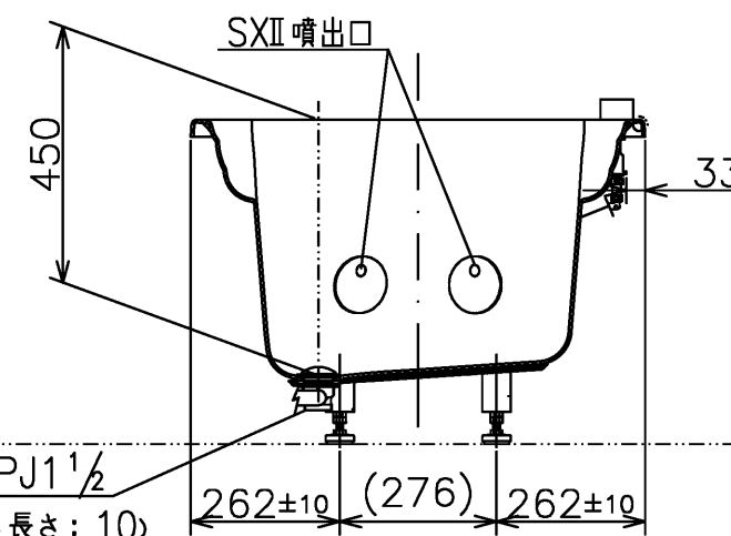
断面A-A
