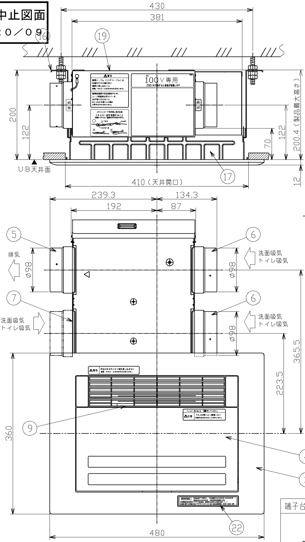
天井取付図 (1:5)
