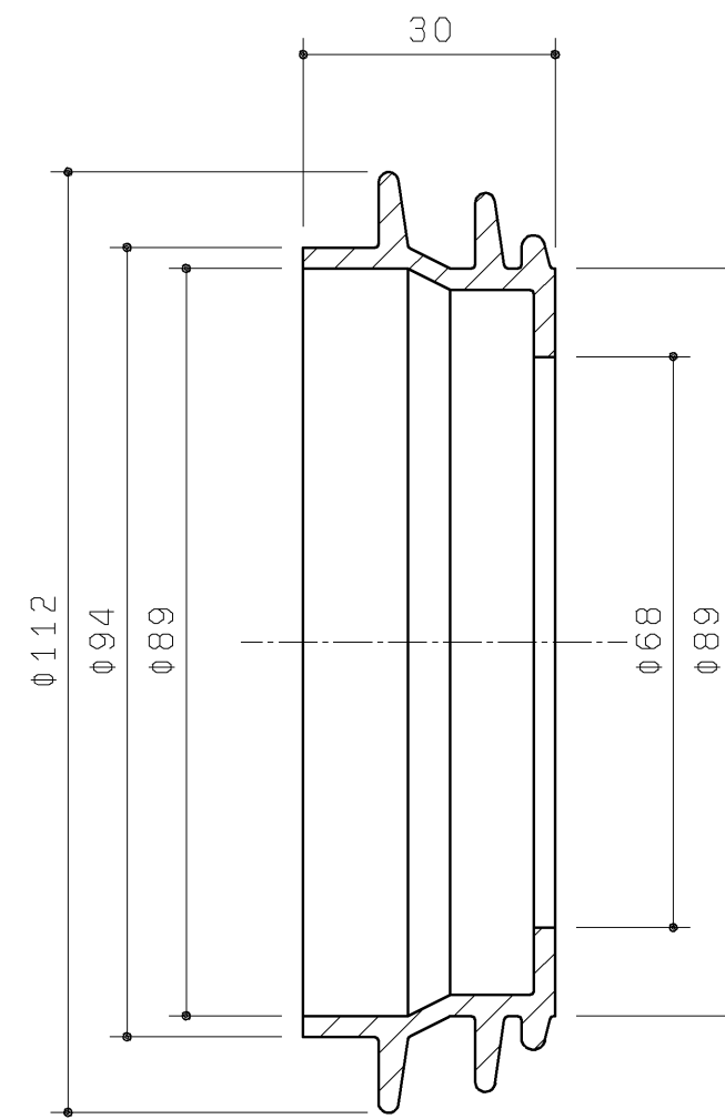
A-A断面図
