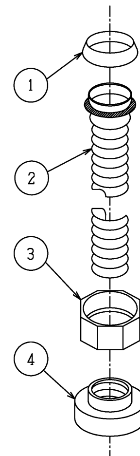
分解図（尺度フリー）
