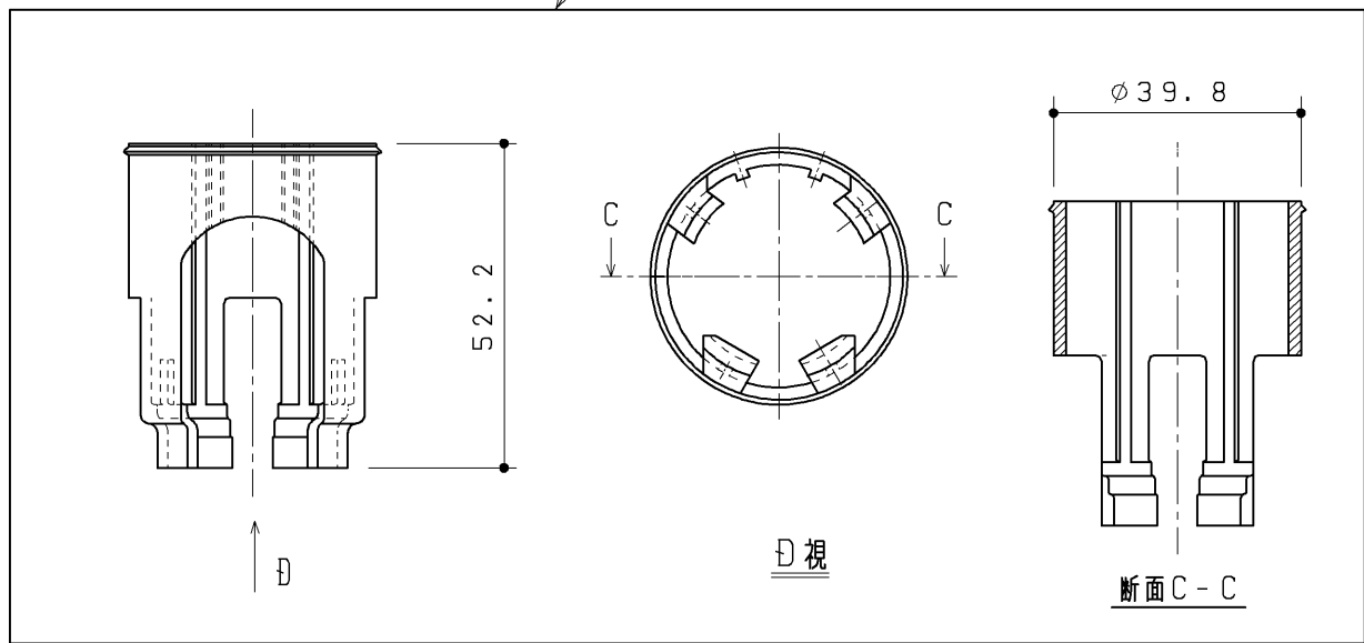
止水栓ハンドル取付材
