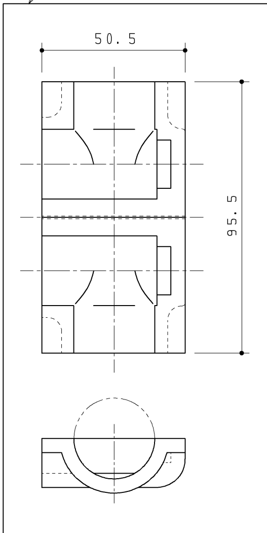
防露材 3ヶ
