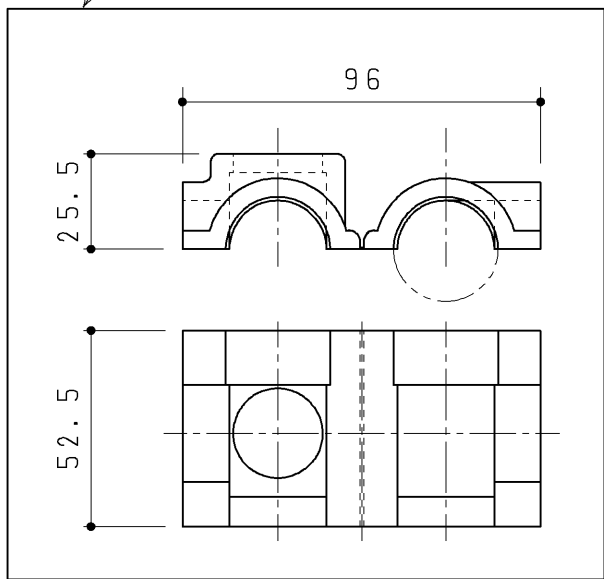
防露カバー（分岐金具部）
