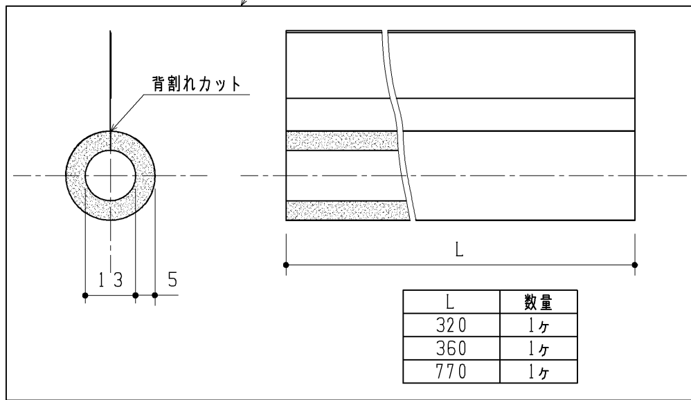
防露材 3ヶ
