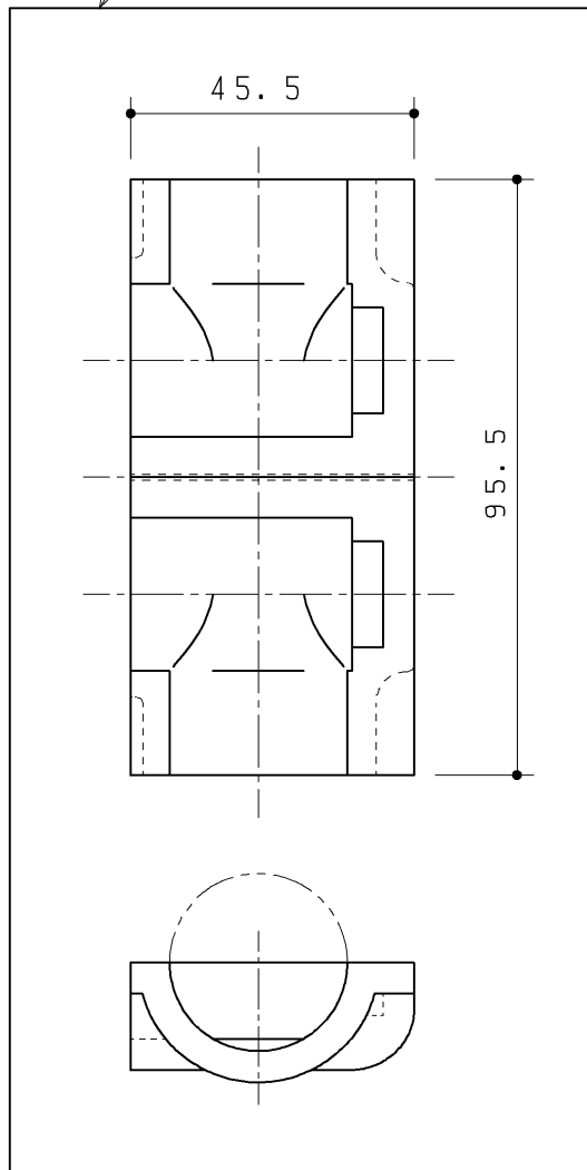
防露カバー（エルボ部）
