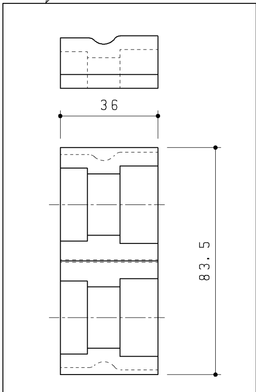
防露カバー（分岐金具部）
