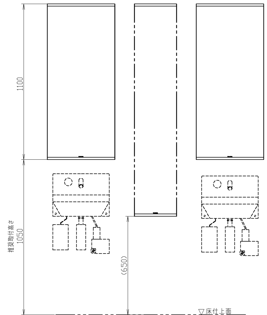
ニューラバトリースペース（棚なし）の場合の推奨取付位置
