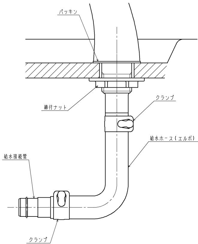
B-B断面詳細図(S=1:1)
