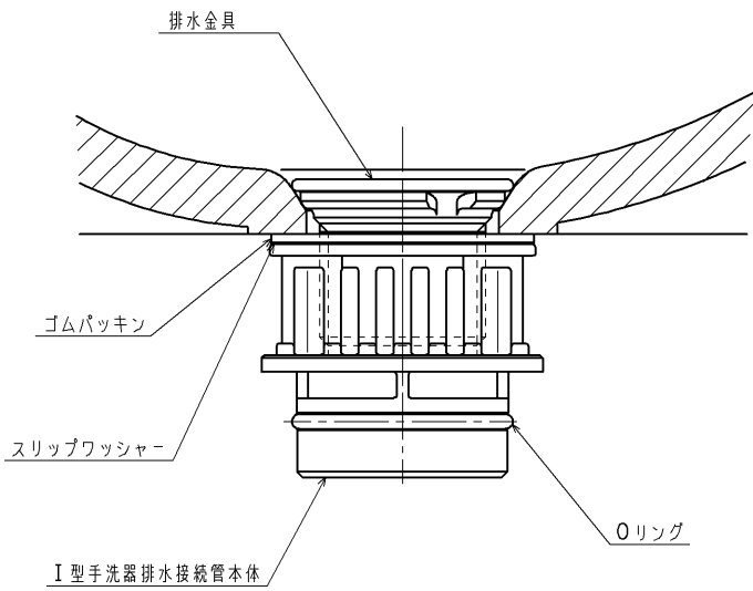
A-A断面詳細図(S=1:1)
