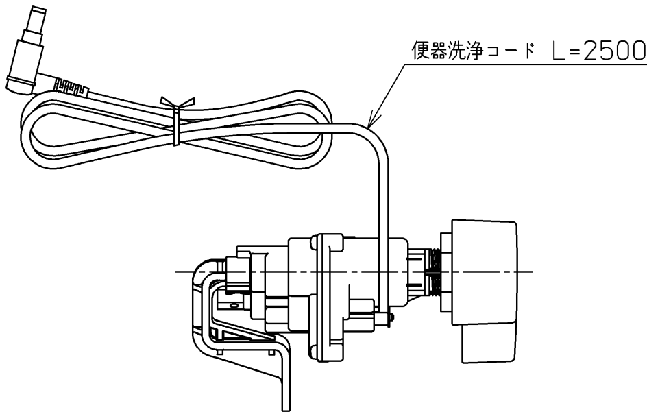
隅付 (C14系・C21系・C416系)
