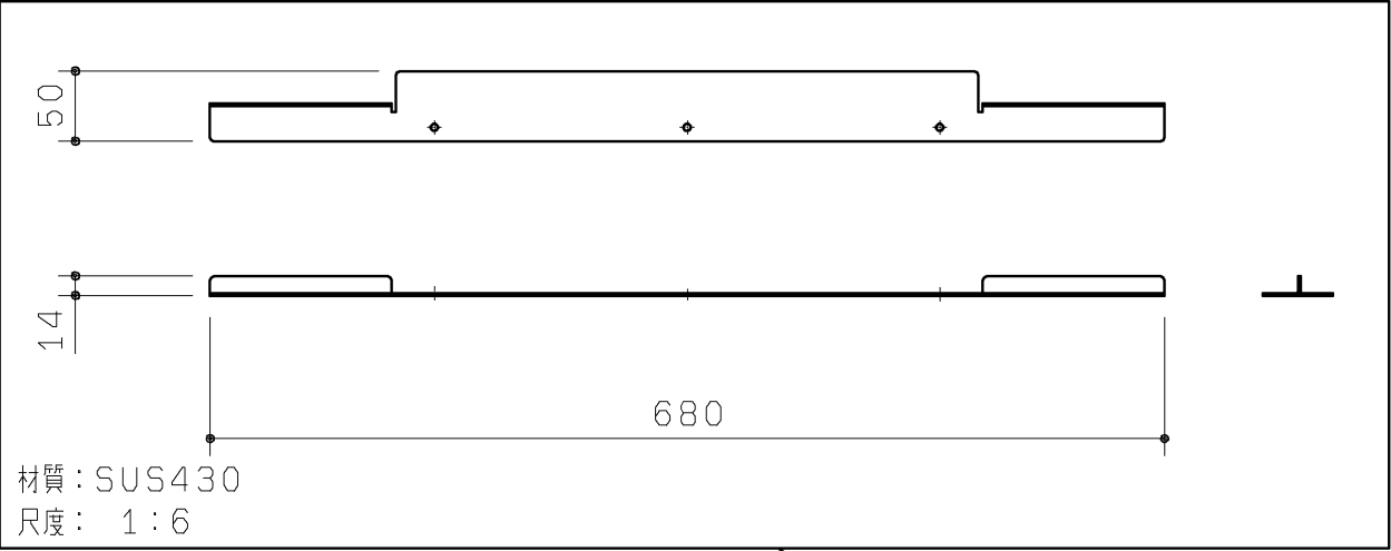
底板支持材
