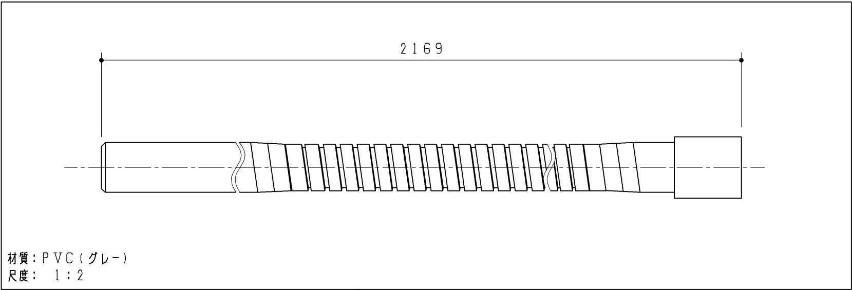
手洗排水ホースセット
