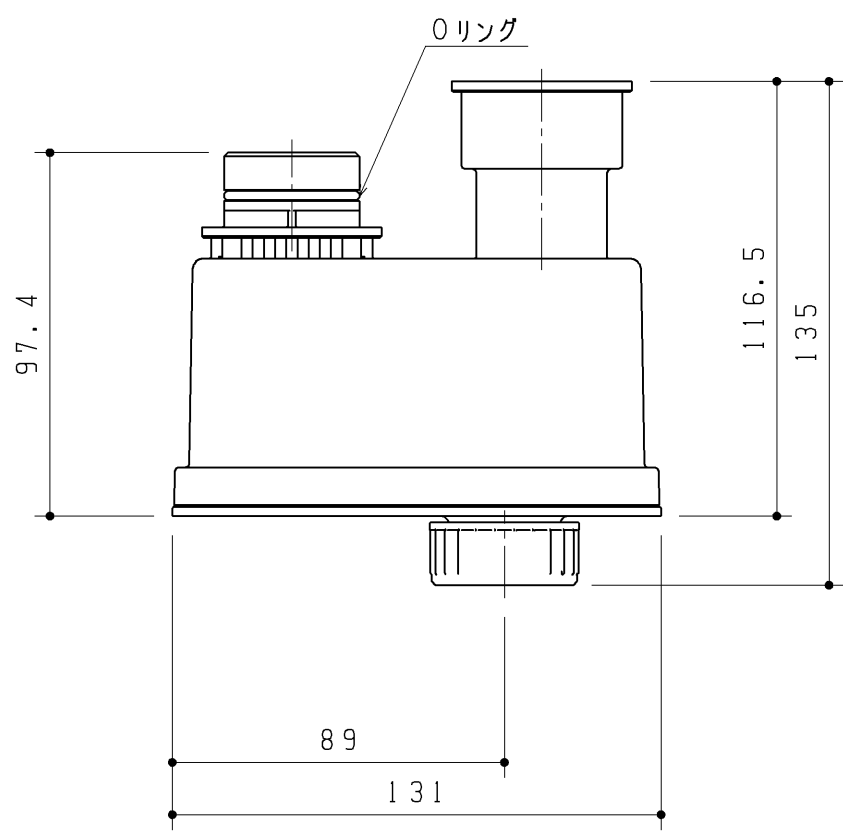
ドラムトラップ (掃除口付)
