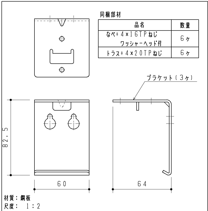
下段カウンター
