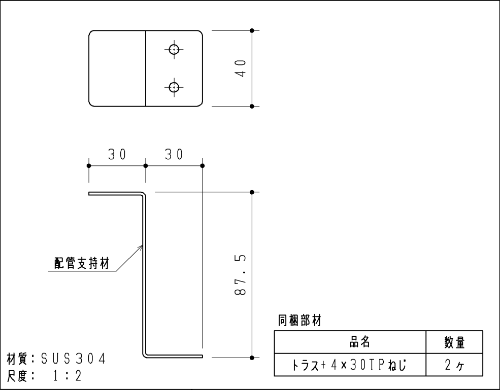
配管支持材セット
