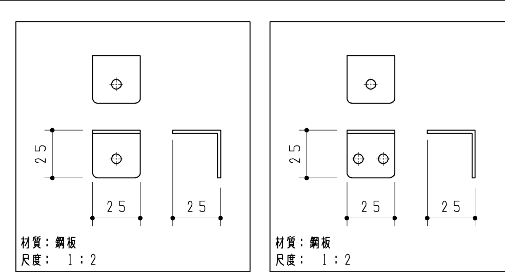
Lアングル
