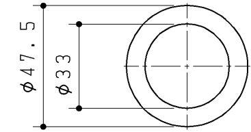
材質：PE (ホワイト) 尺度： 1 : 2
