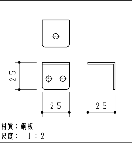
アングル材
