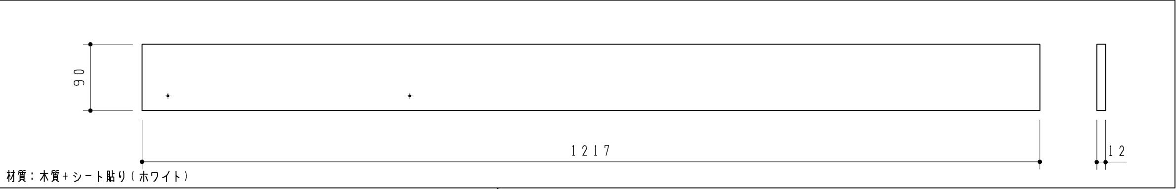
上段補強桟
