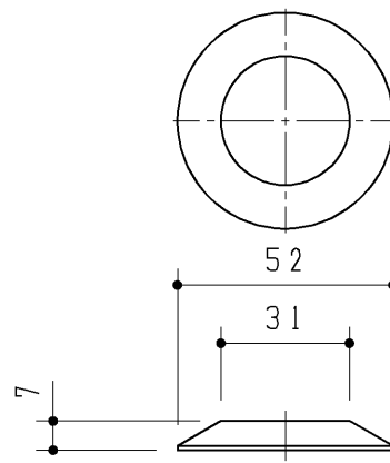
トラップ接続管
