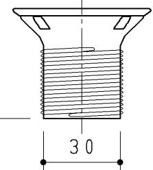
材質：PP (ホワイト) SUS 304 (光沢仕上げ) 尺度： 1 : 2
