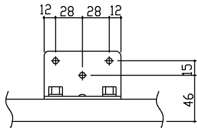
壁固定位置詳細（1／10）
