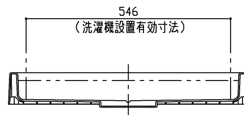
断面B-B
