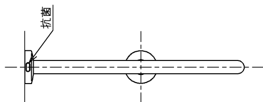
取付座詳細(1:2)
