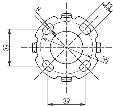
取付座詳細(1:2)
