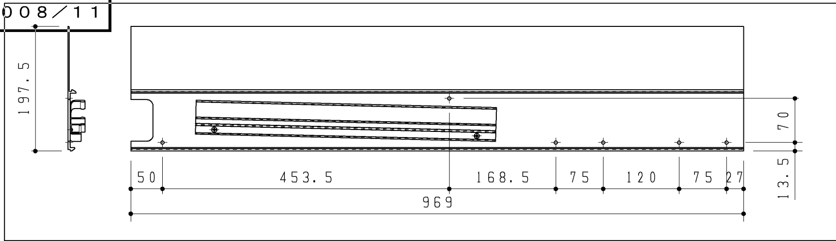
配管カバー
