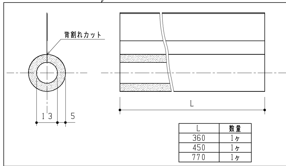
防露材 3ヶ
