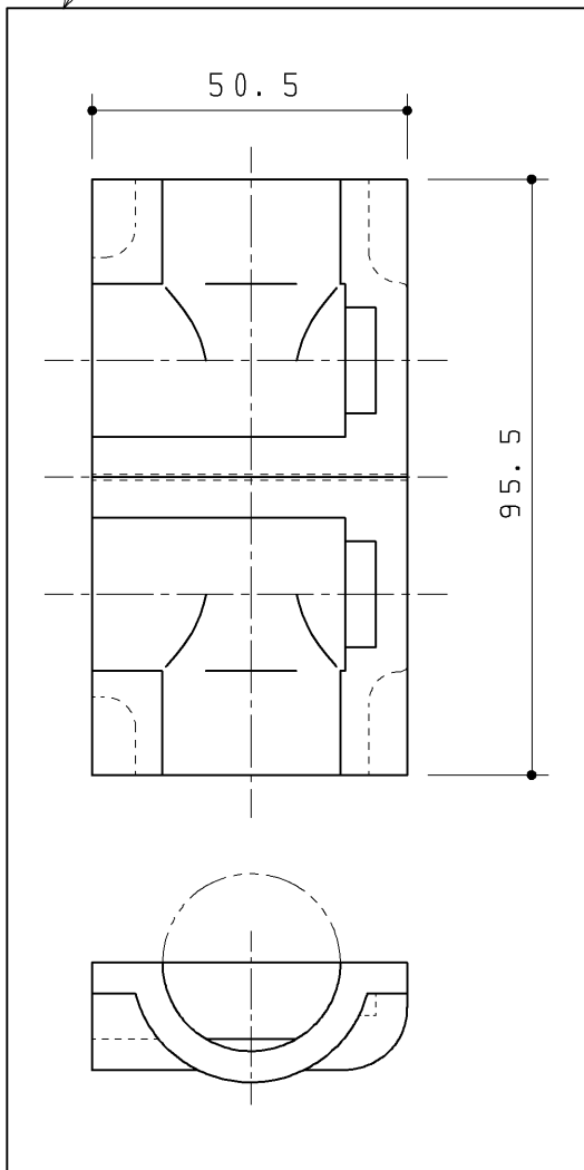
防露材 3ヶ
