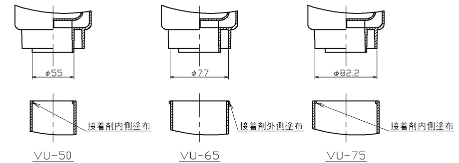
適合排水管（VU-50、VU-65、VU-75）尺度1:5
