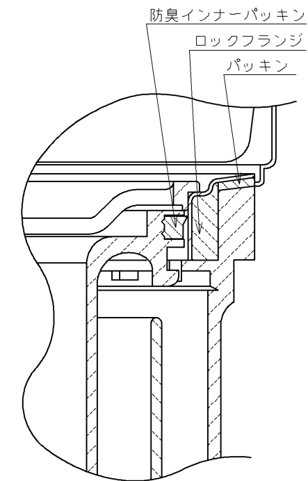
C部詳細図（縮尺 1：1）
