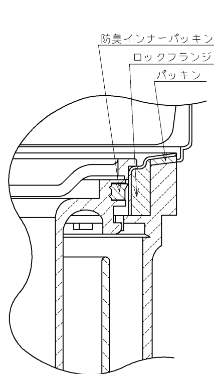
C部詳細図(1:1)
