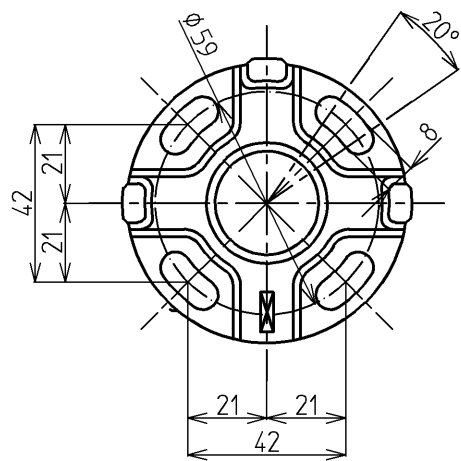
取付座詳細(1:2)
